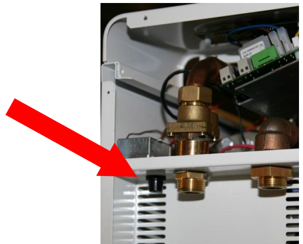
Situación del limitador en una caldera CM sólo calefacción.
